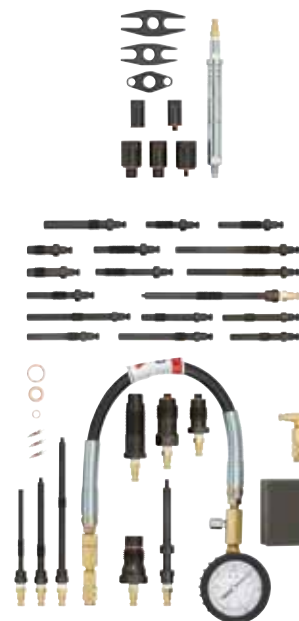
Art. 818010 Set prova compressione Master, 37 pezzi
