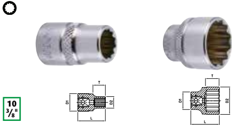
CHIAVE A BUSSOLA 3/8", 12 PT. DIN. 3120
