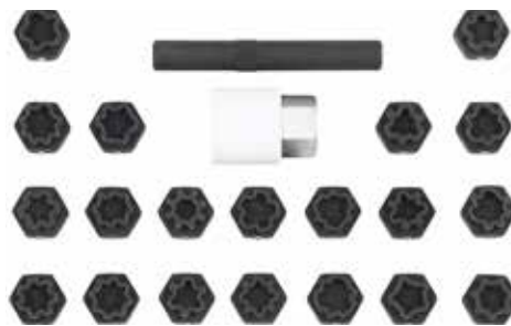
Art. 829006 Set chiavi a stella per ruote - Audi, 22 pezzi Set audi completo comprendente adattatore da 21 mm con azionamento quadrato da 1/2" questo kit è progettato per la rimozione dei bulloni di bloccaggio quando il cliente si è dimenticato di lasciare l'adattatore sull'auto. Ciò succede frequentemente quando il veicolo viene portato a riparare e/o lo si sottopone a manutenzione. Adatto per oem T40073.
