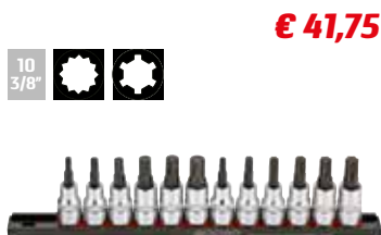
Art. 201201 Set di chiavi a bussola a giravite ribe e triple square 3/8", su binario 12 pezzi - Spline M5, M6, M8, M9, M10, M12 - Ribs M5, M6, M7, M8, M9, M10
