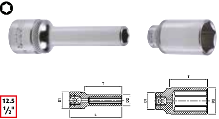
CHIAVE A BUSSOLA PROFILO FLANK 1/2" LUNGA, 6 PT. DIN. 3120/3124
