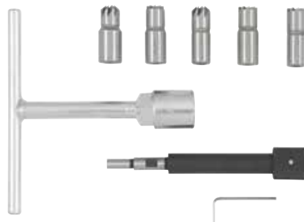
Art. 818004 Set per pulizia sedi iniettori, 7 pezzi
