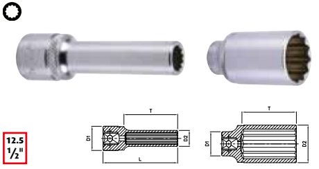
CHIAVE A BUSSOLA 1/2" LUNGA, 12 PT. DIN. 3120
