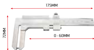
Art. 47024 Calibro a corsoio per disco freni in acciaio inox
