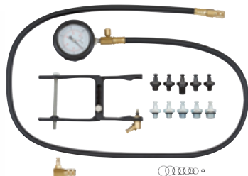
Art. 818011 Set di prova pressione dell'olio, 14 pezzi
