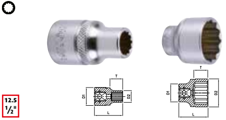
CHIAVE A BUSSOLA 1/2", 12 PT. DIN. 3120
