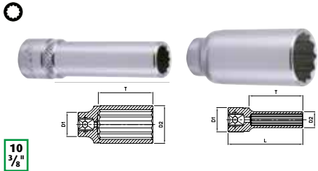
CHIAVE A BUSSOLA 3/8" LUNGA, 12 PT. DIN. 3120
